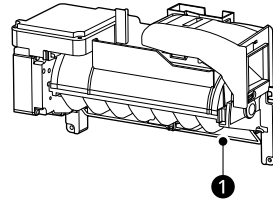
❶ Arrêt automatique (bras palpeur)
