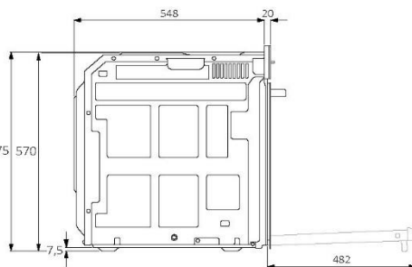
Vista laterale
