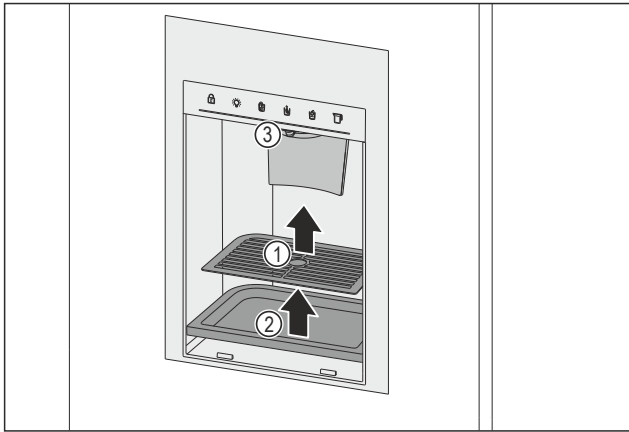
Fig. 150 Retrait de la grille d'écoulement et du bac d'écoulement
