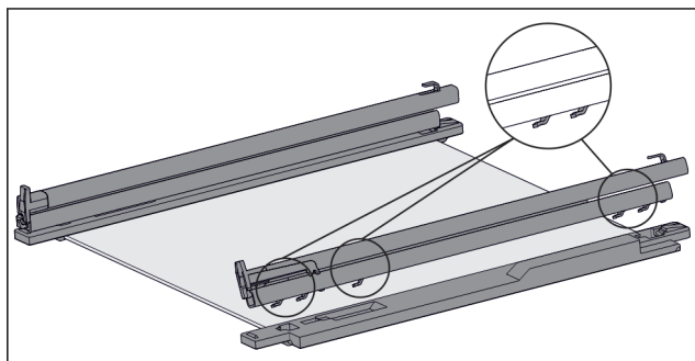
Fig. 34 Tablette en verre avec rails et pièces de retenue
