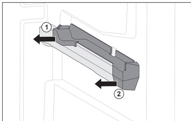
Fig. 31 Élément emboîtable sur la nervure de récipient droite
