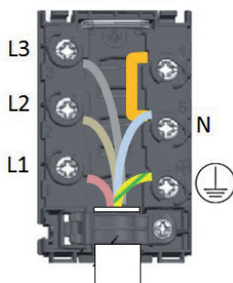
400V~ 3P+N
