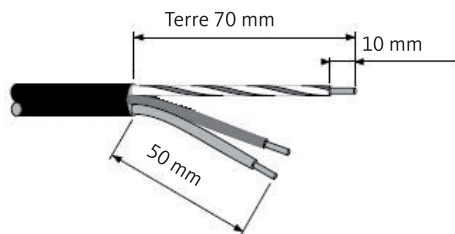
Extrémité du câble d'alimentation
