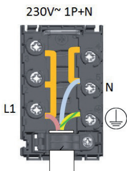
Branchement d'usine
