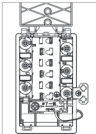
400V~ 3P+N
