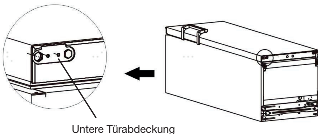
Untere Türabdeckung
