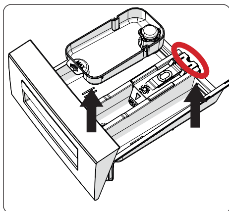
Siphon adoucissant(*)
